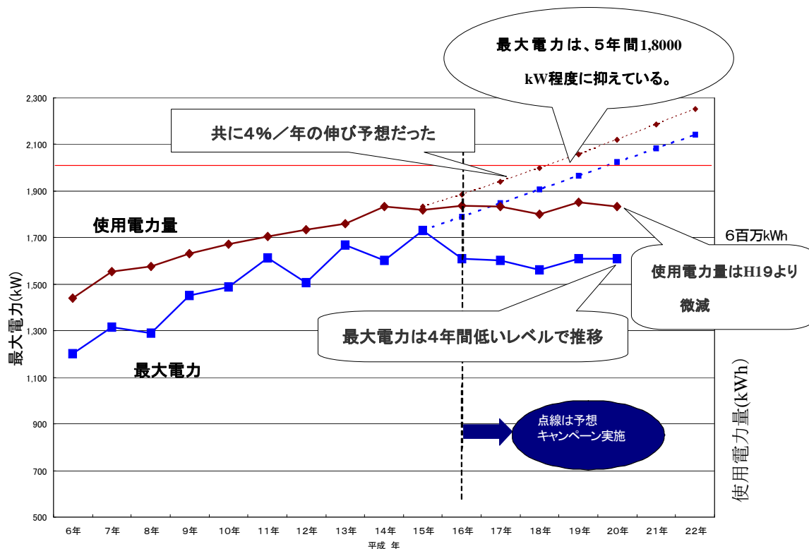
品川キャンパス 最大電力と使用電力量
